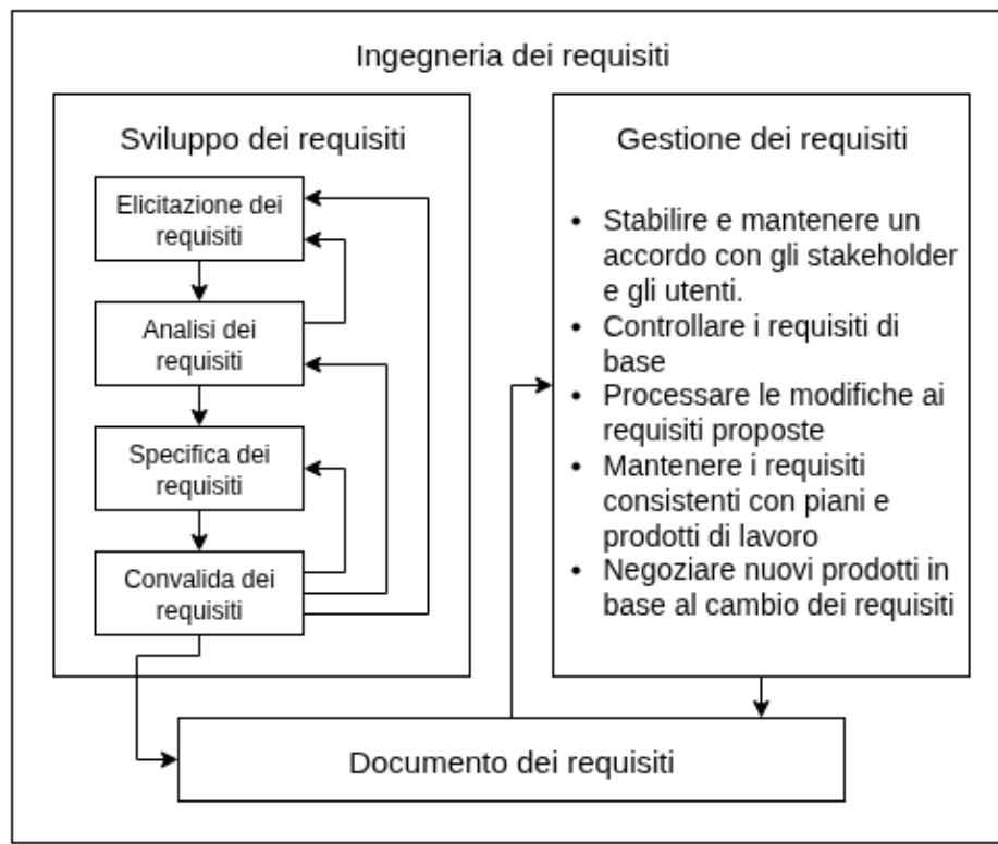
Figura 3.1: Processi dell'ingegneria dei requisiti
