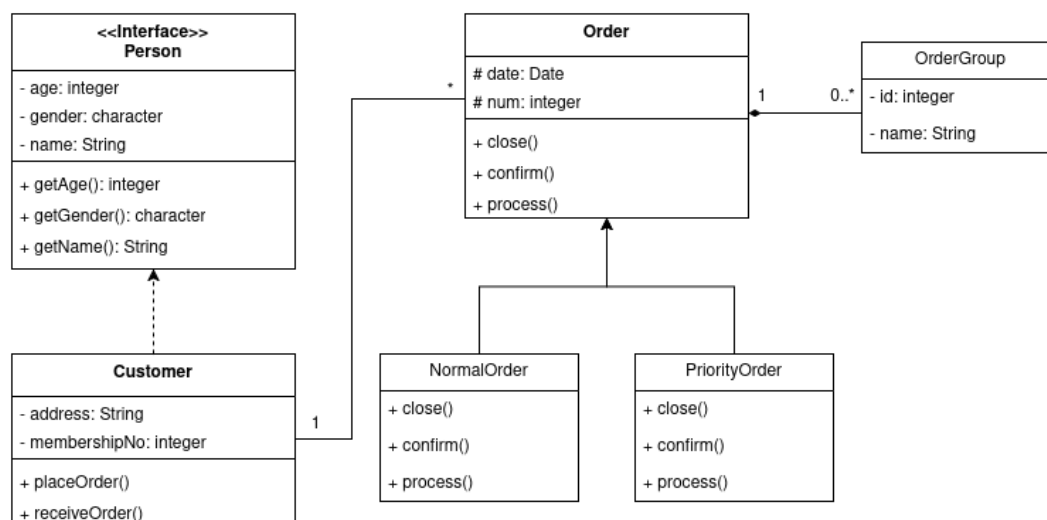
Figura 5.2: Esempio class diagram
