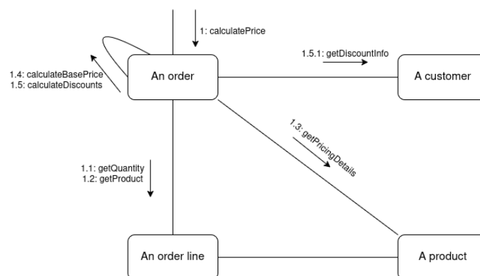
Figura 5.5: Esempio communication diagram
