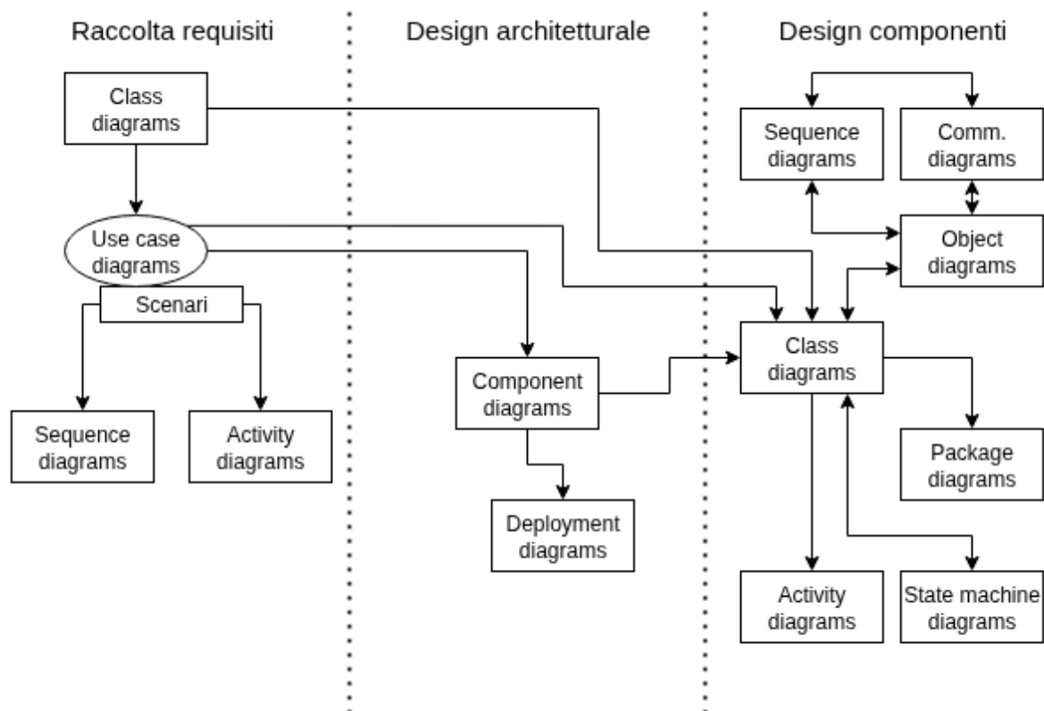
Figura 5.1: Panoramica diagrammi UML 2.0
