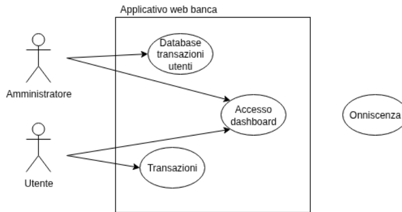
Figura 3.2: Esempio di use case diagram
