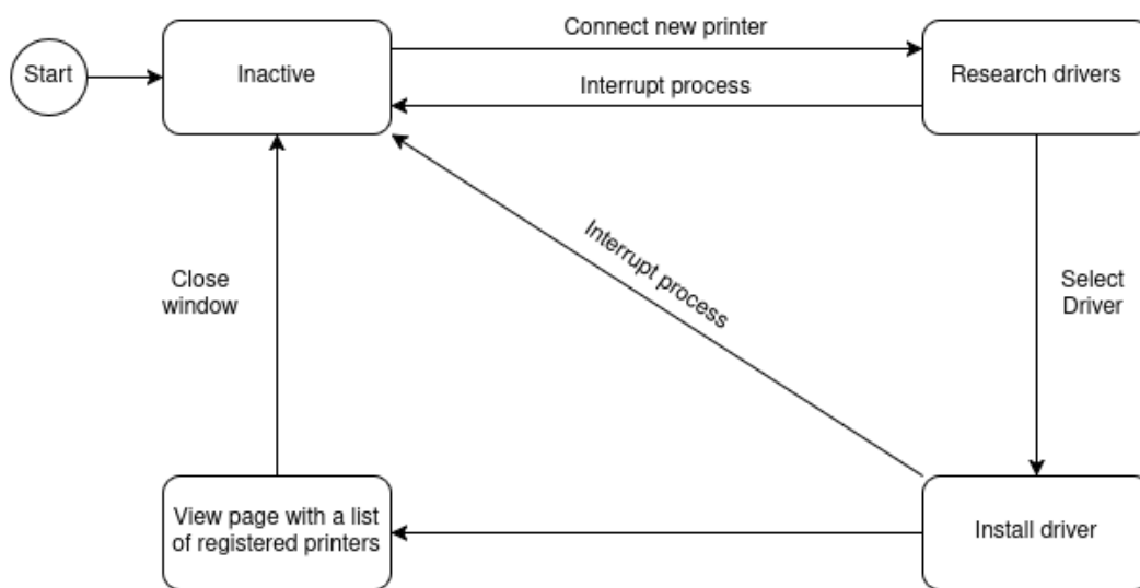
Figura 5.6: Esempio state machine diagram
