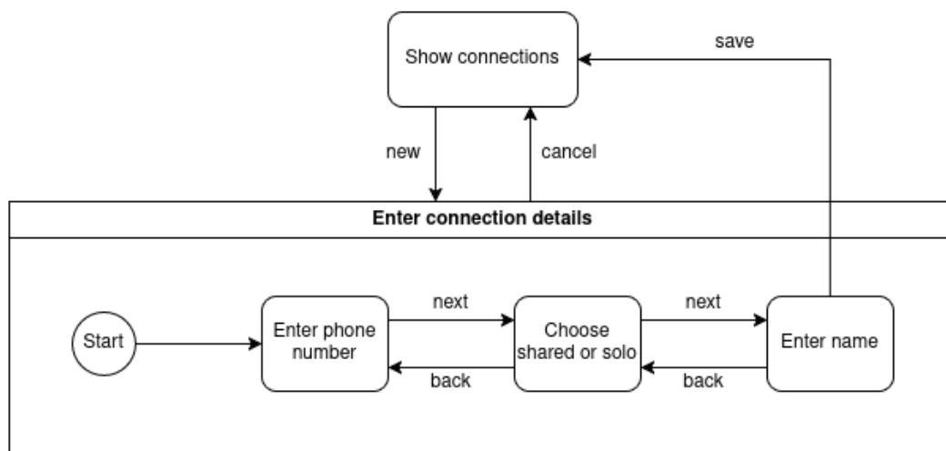
Figura 5.7: Esempio stato composito
