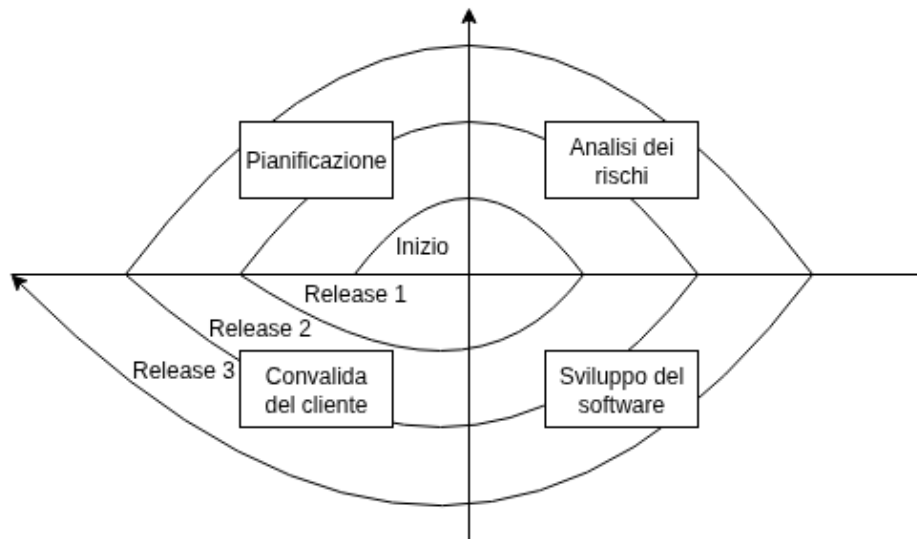
Figura 2.3: Modello a spirale
