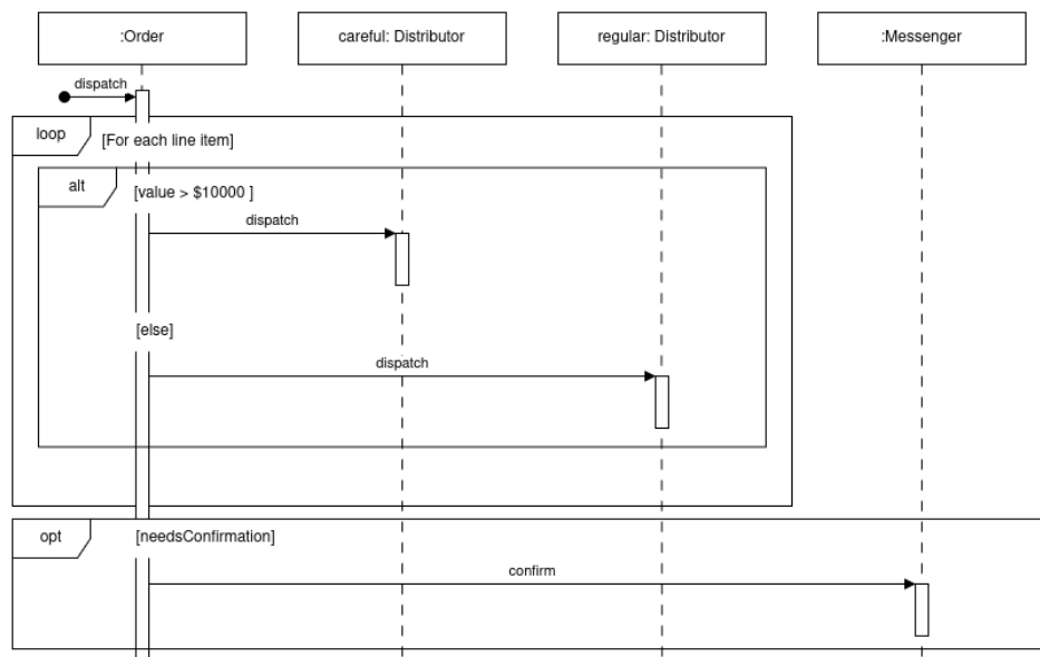
Figura 5.4: Esempio sequence diagram
