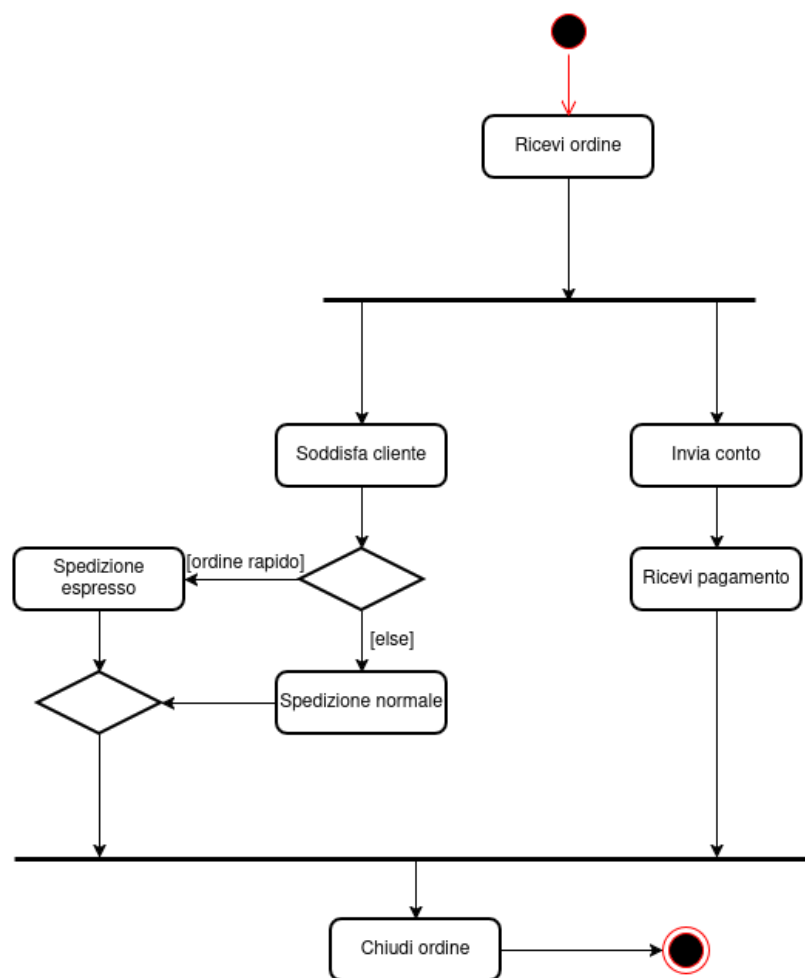
Figura 5.8: Esempio activity diagram
