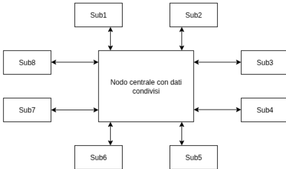
Figura 4.2: Modello repository
