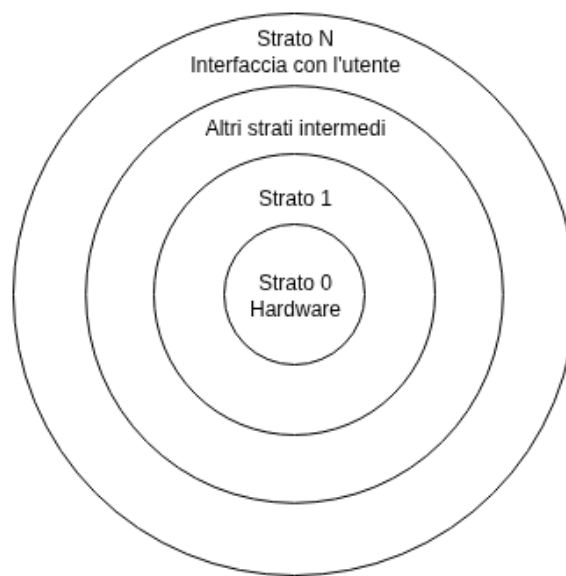
Figura 4.1: Modello stratificato
